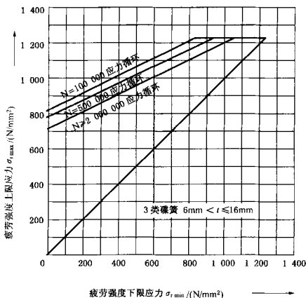
图 C.11 6 mm < t \leq 16 mm 碟簧的疲劳强度曲线图
